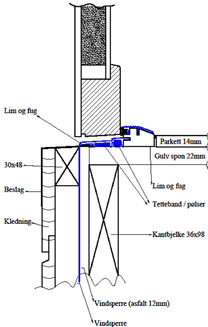
Prinsipp-skisse for å tette under terskel Balkong / ytterdør
